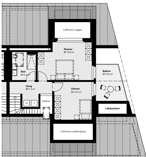
2. Dachgeschoss
