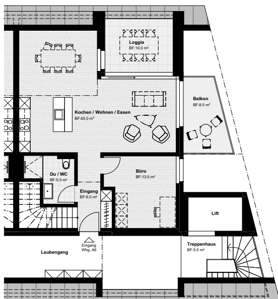
1. Dachgeschoss
